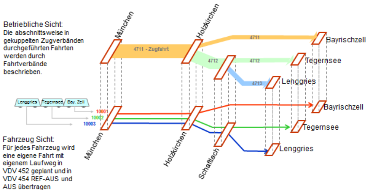
Abbildung 48 Beispiel "Flügelbetrieb"
