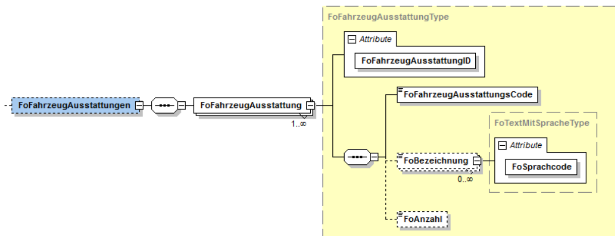
Abbildung 7 Element "FoFahrzeugAusstattungen"
