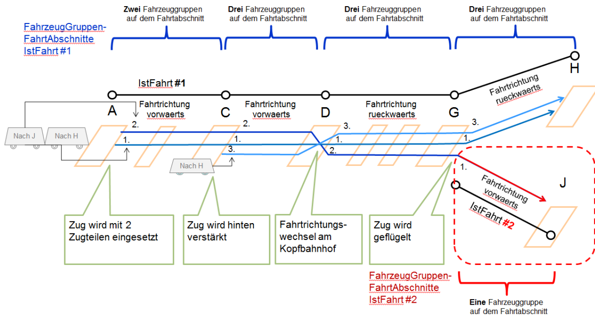
Abbildung 14 Beispiel Fahrtabschnitte
