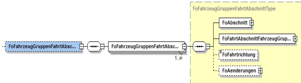
Abbildung 13 Element "FoFahrzeugGruppenFahrtAbschnitte"
