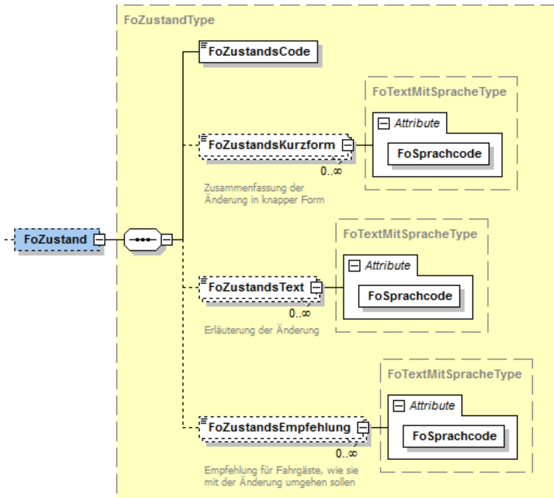
Abbildung 46 Element "FoZustand"
