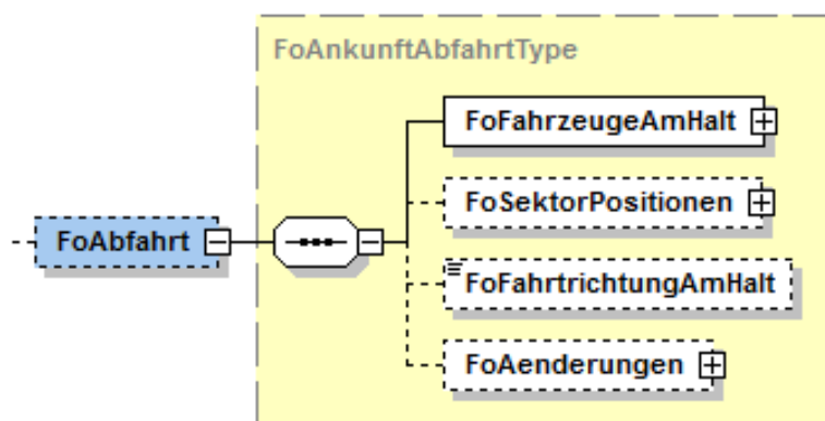
Abbildung 37 Element "FoAbfahrt"
