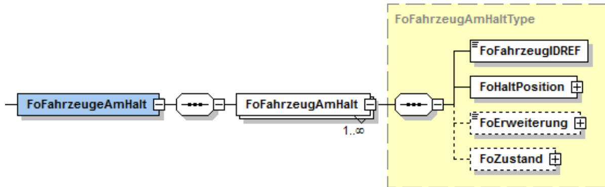
Abbildung 33 Element "FoFahrzeugeAmHalt"
