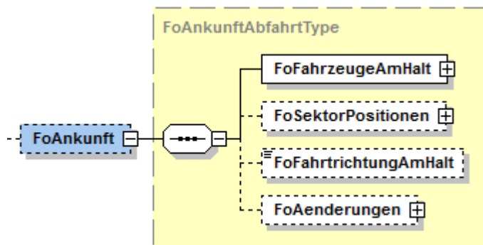
Abbildung 32 Element "FoAnkunft"
