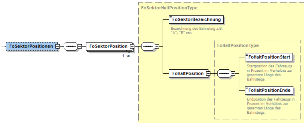
Abbildung 40 Element "FoSektorPositionen"
